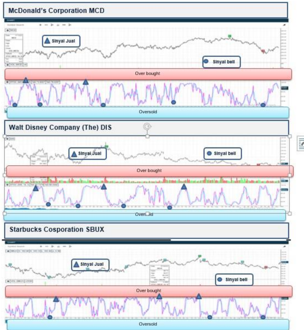
Gambar.3 Teknikal Stochastic
