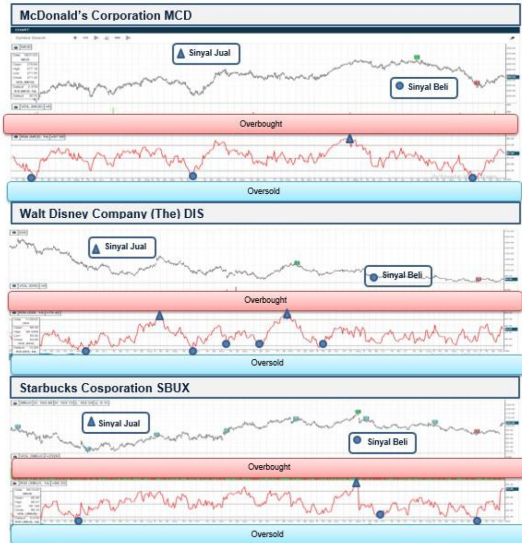
Gambar.4 Teknikal RSI
