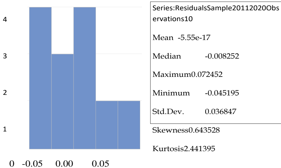
Gambar 1. Uji Normalitas
