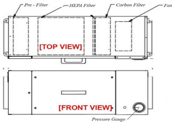
Gambar 2. Gambaran Exhaust Fan
